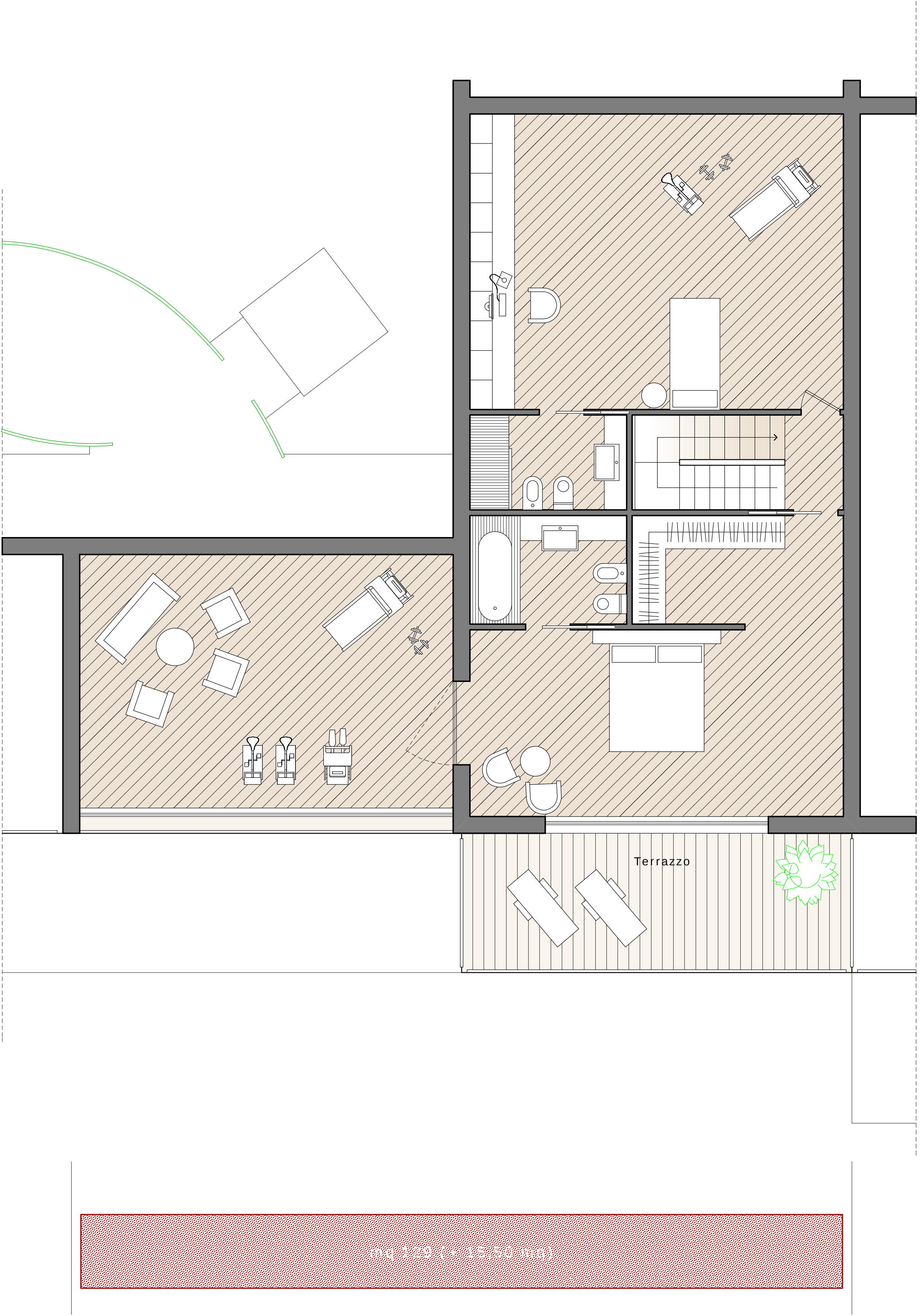
LIVELLO SOTTOTETTO Scala 1:50
