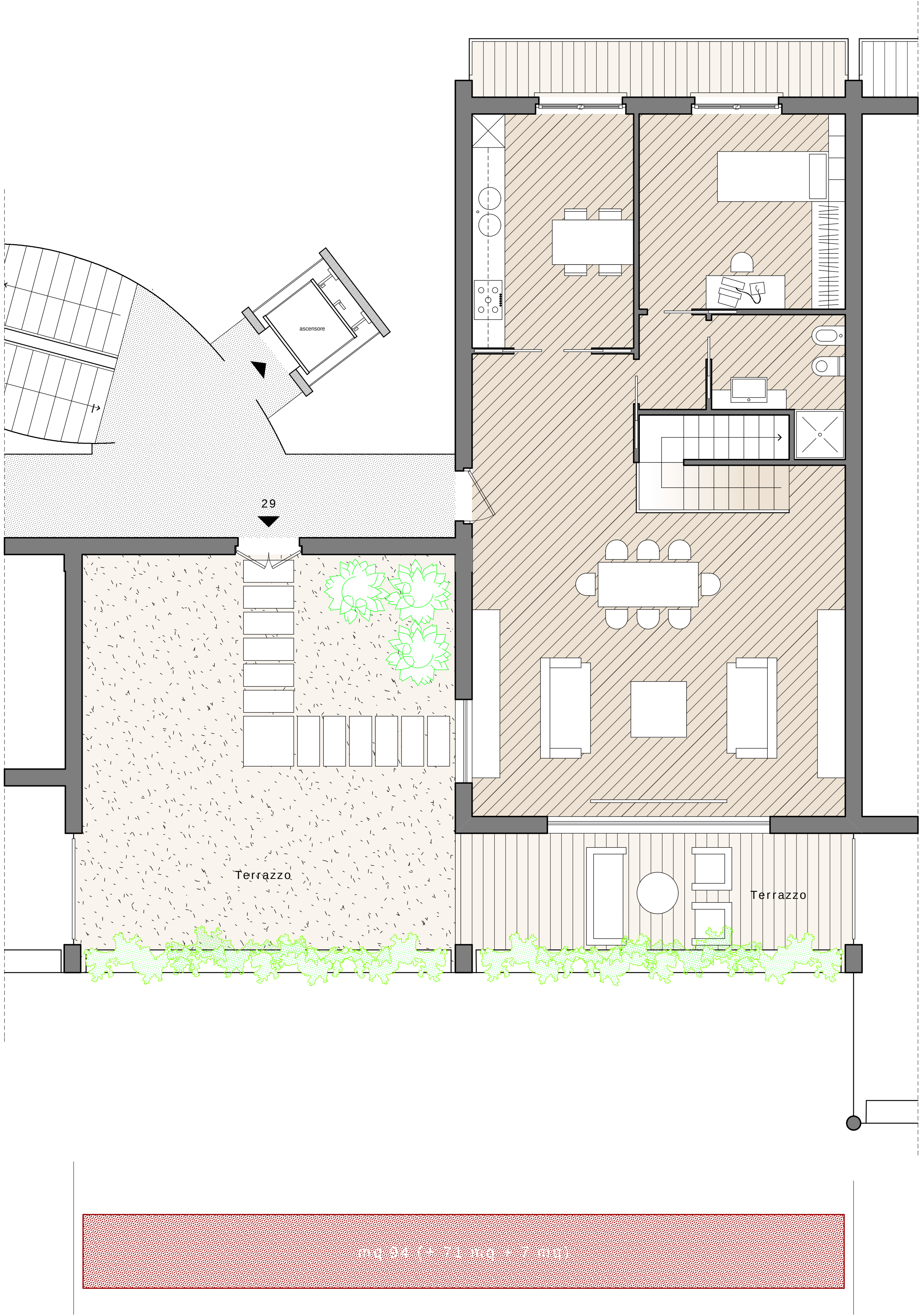
LIVELLO +5 Scala 1:50
